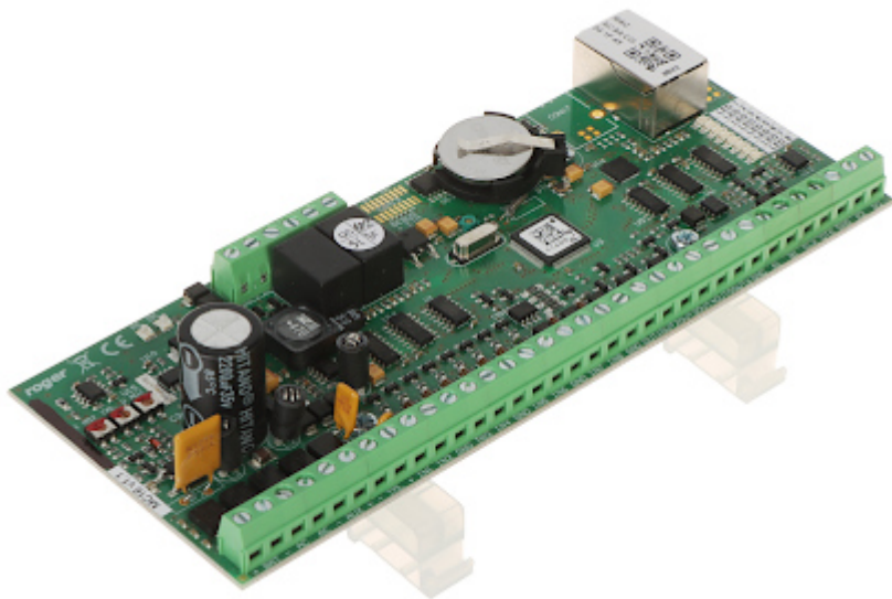
Изглед отгоре:
